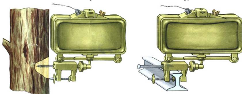
Установка мины на деревянных и металлических конструкциях
