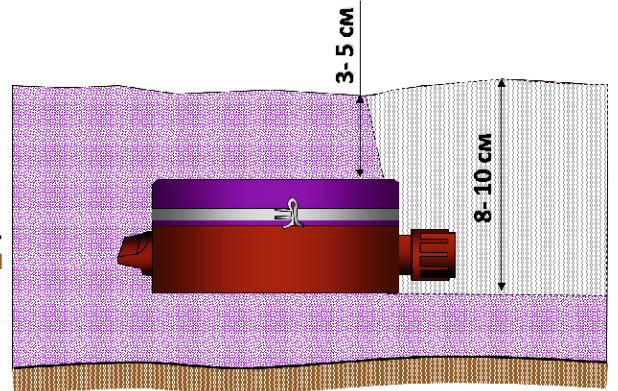
Установка мины ПМН в рыхлый снег
